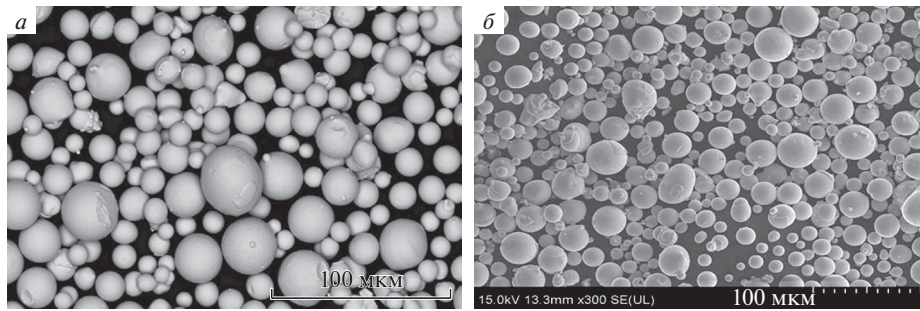
Рис. 2. Металлопорошковая композиция Metco 68F-NS-1 производства ОС Oerlikon Corporation AG (а) и металлопорошковая композиция Co–Mo–Cr производства НИЦ “Курчатовский институт” – ВИАМ (б)
